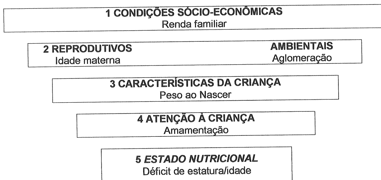
Figura 1: MODELO TEÓRICO
